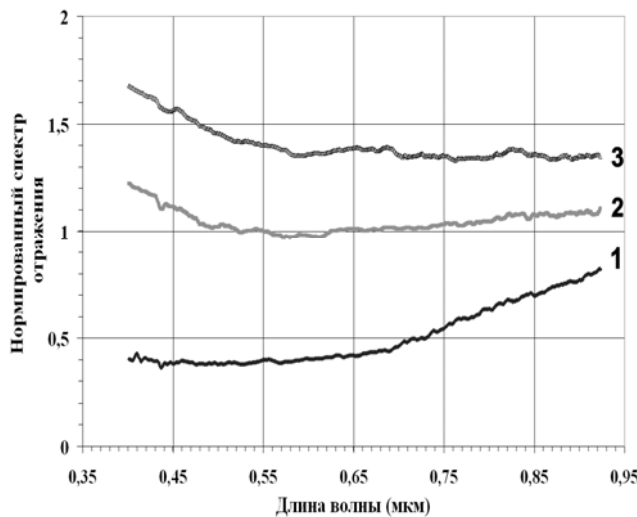
Рис. 3. 21 Лютеция (05/06-11-04)
